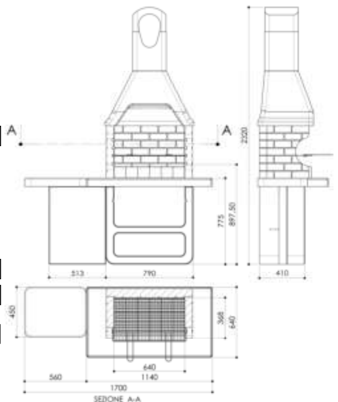
Vooraanzicht met maataanduiding
