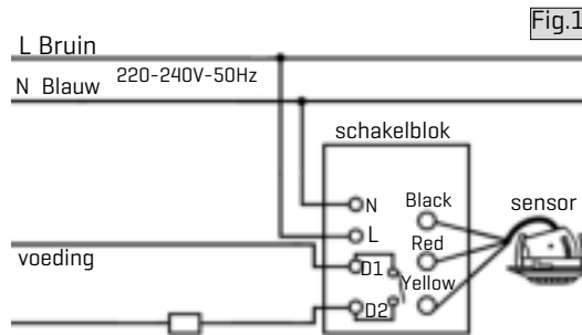
Fig 1+2: aansluitschema's
