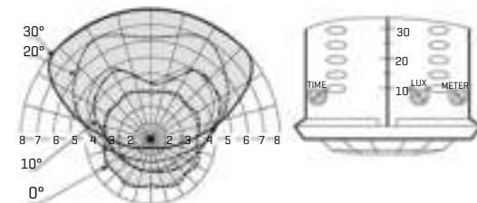
Fig.6: detectieveld
