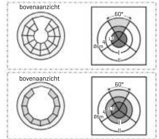
Fig.6: detectieveld
