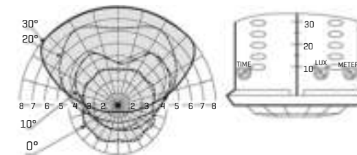
Bild 6: Detektionsbereich
