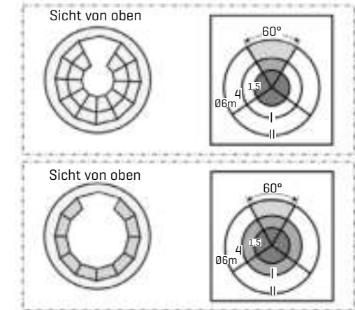
Bild 6: Detektionsbereich
