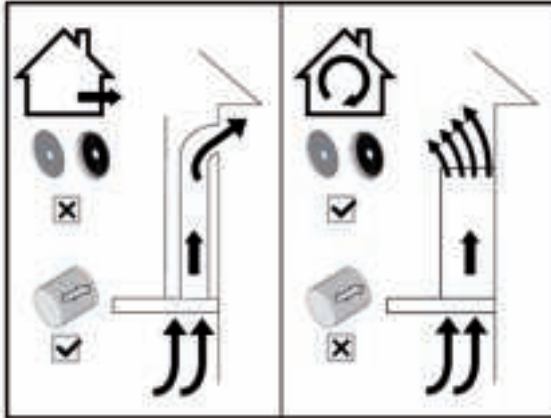
Fonction extraction
