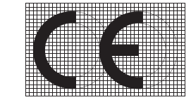
CE标志, 请严格按照此网格比例来制作 在印刷件上显示最小高度为5MM(等比例缩放)
