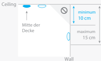
Abbildung 4 Optimale und akzeptable Positionen für Rauchmelder
