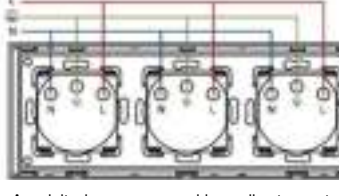
Aansluitschema van een drievoudig stopcontact (II)
