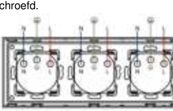
Aansluitschema van een drievoudig stopcontact (I)
