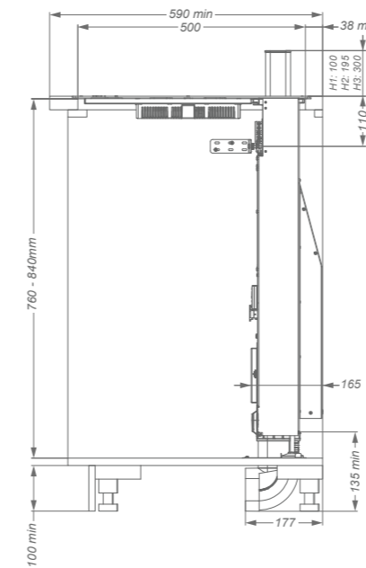
Zijaanzicht
