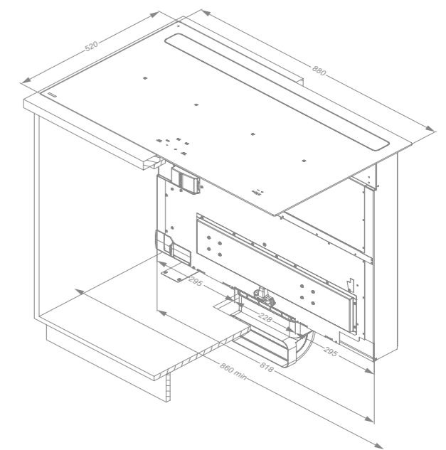
3D tekening
