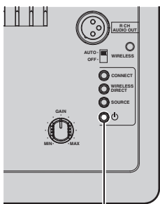
Linker Lautsprecher (Rückseite)
