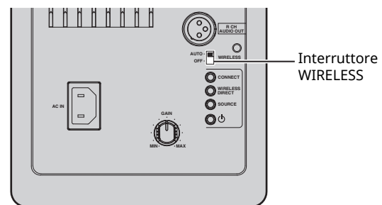
Diffusore sinistro (pannello posteriore)
