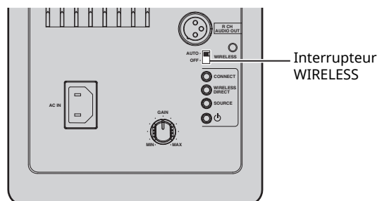
Enceinte gauche (face arrière)
