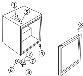
Fig 2 Positie van de onderdelen na het omdraaien van het deurscharnier.
