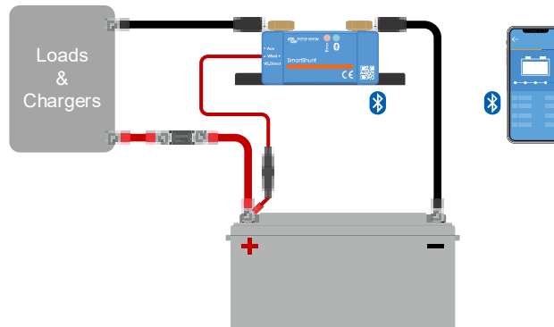
Standaard SmartShunt-bedrading
