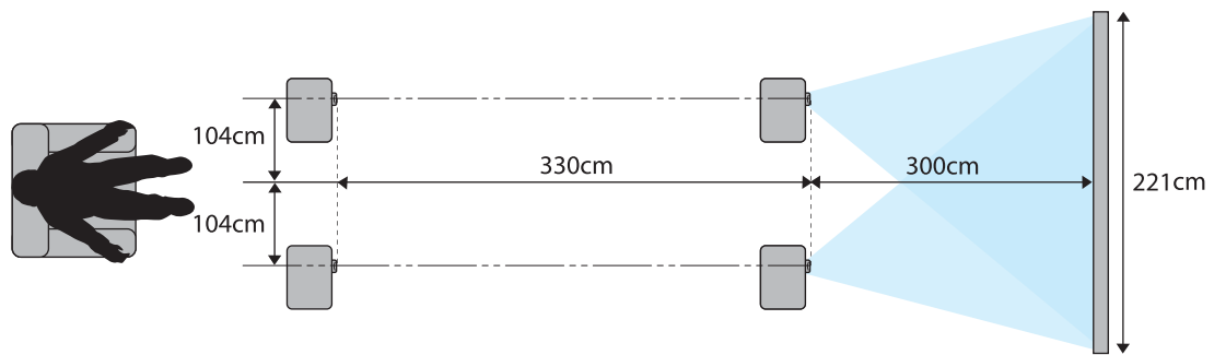
Bovenaanzicht
