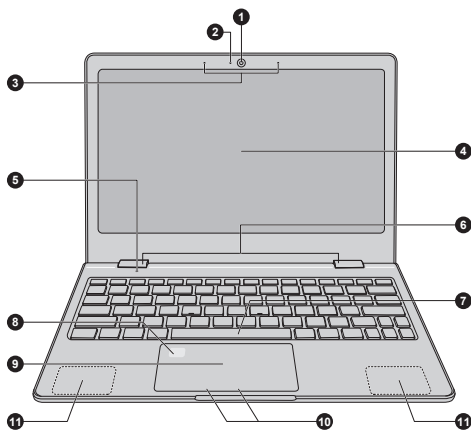
Afbeelding 3-5 Voorkant van de computer met geopend beeldscherm
