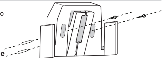
Figura 2 Fissaggio del supporto di ricarica alla parete
