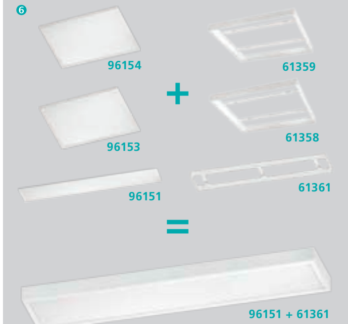
6 OPBOUWARMATUUR FRAME SURFACE LUMINAIRE RAHMEN AUFBAULEUCHTE LUMINAIRE EN SAILIE AVEC BOX
