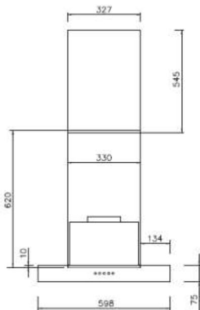
Vooraanzicht
