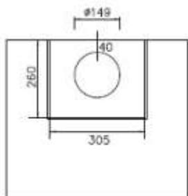
Bovenaanzicht
