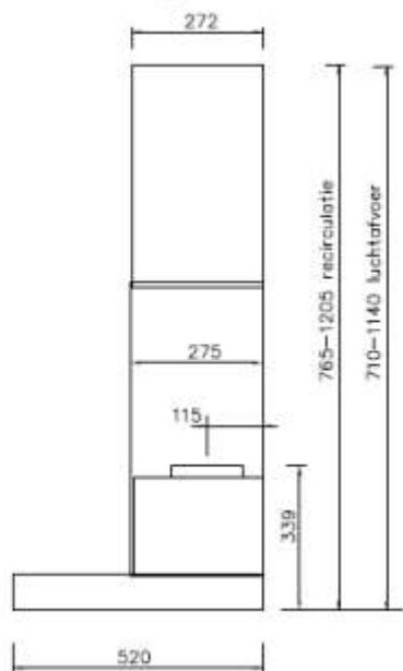
Rechter zijaanzicht
