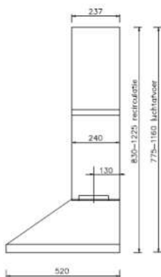
Rechter zijaanzicht
