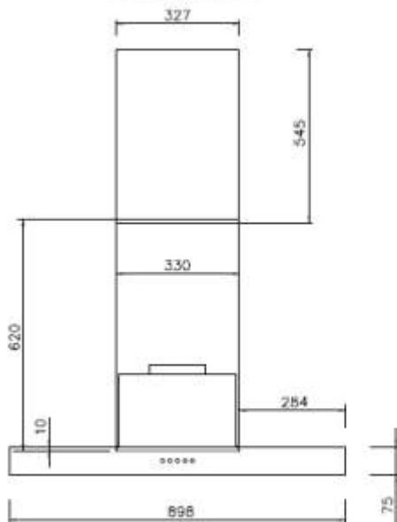
Vooranzicht
