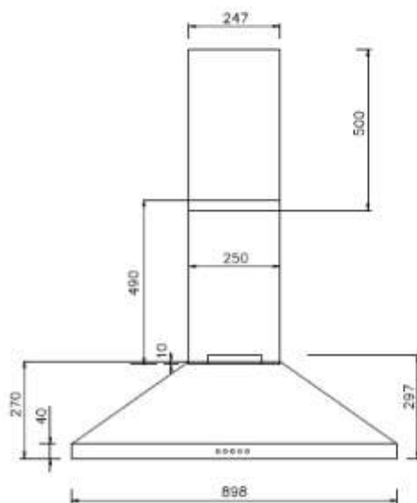
Vooranzicht
