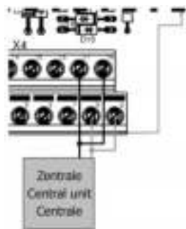
Fig. 2: Stroomtoevoer via de centrale
