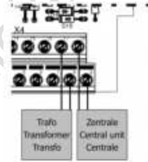
Fig. 3: Stroomtoevoer via een aparte trafo
