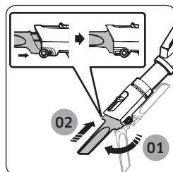
6 Sprekkverktøy
