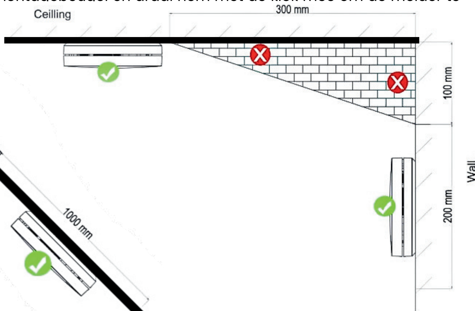
Figuur 4: Aanbevolen montagelocaties
