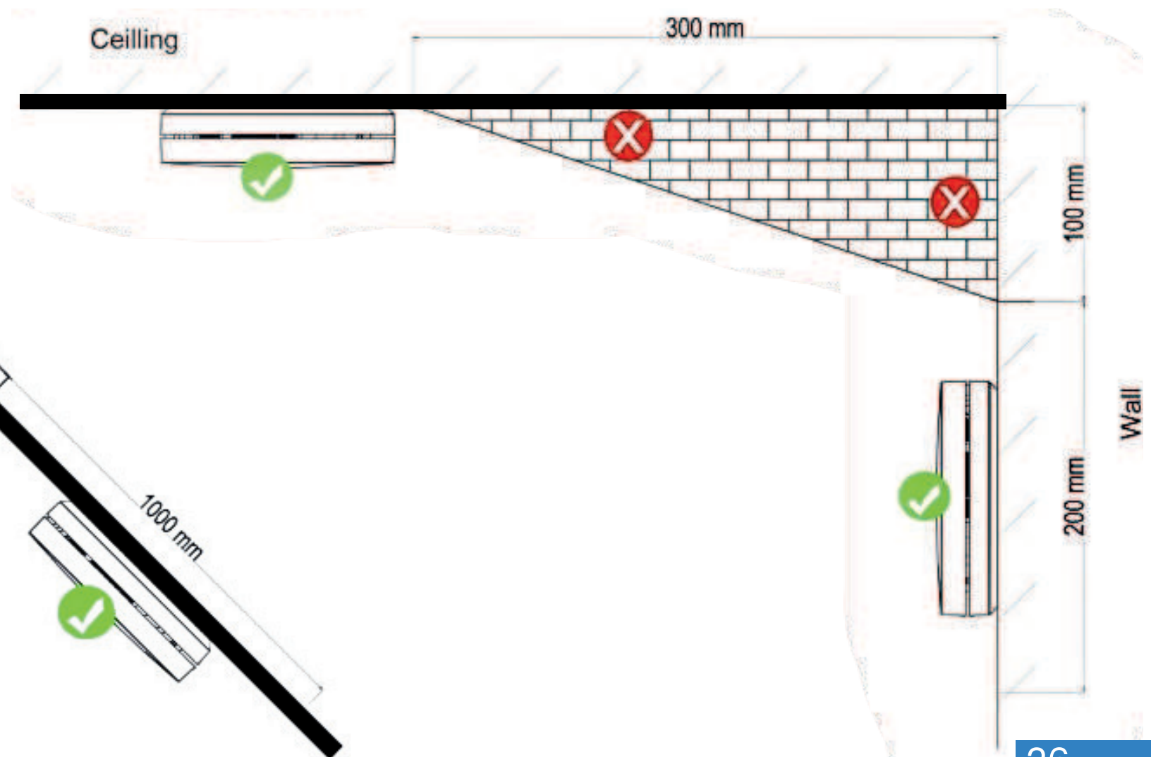
Figura 5: posizioni di montaggio consigliate
