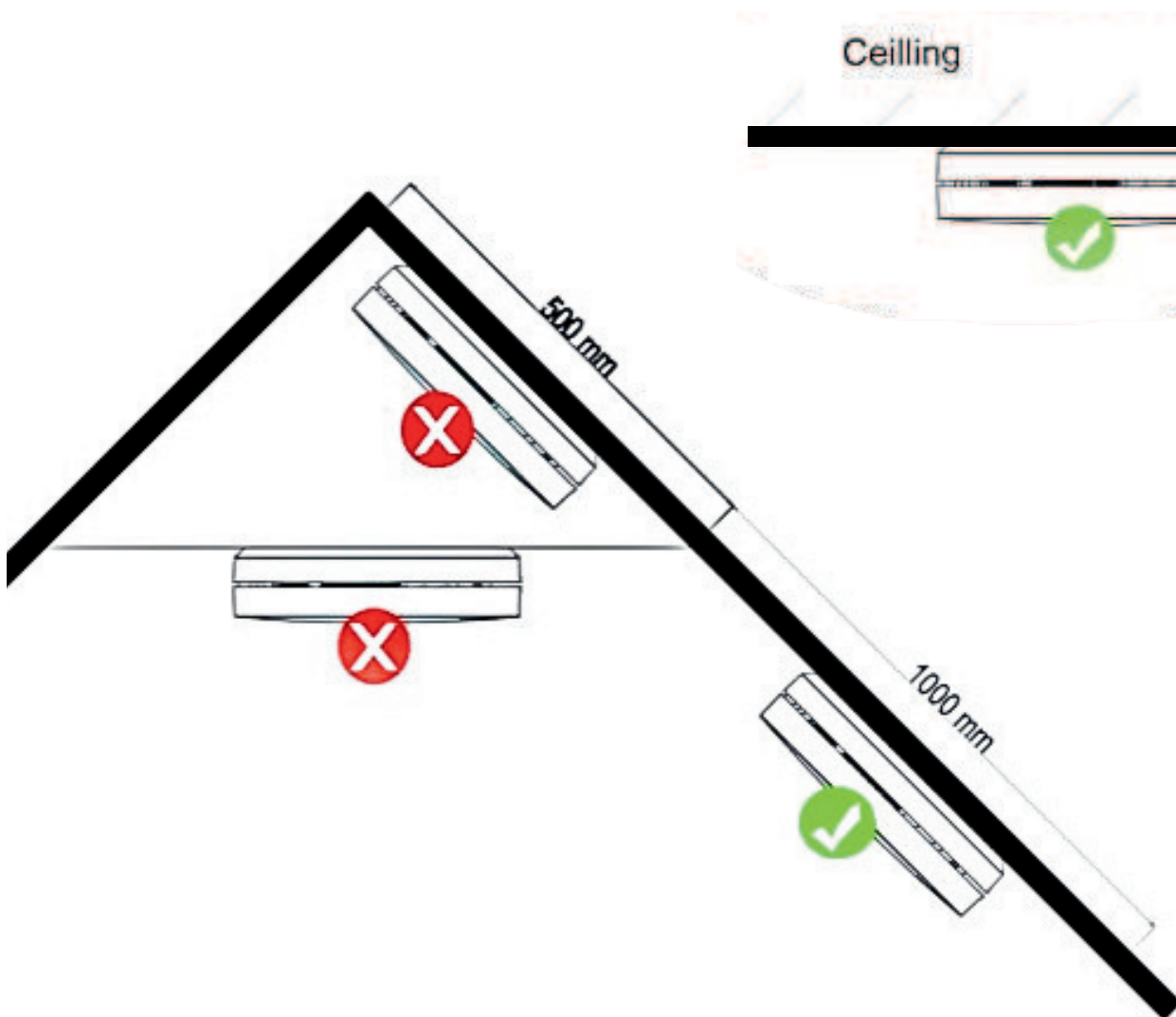
Figura 4: posizioni di montaggio consigliate
