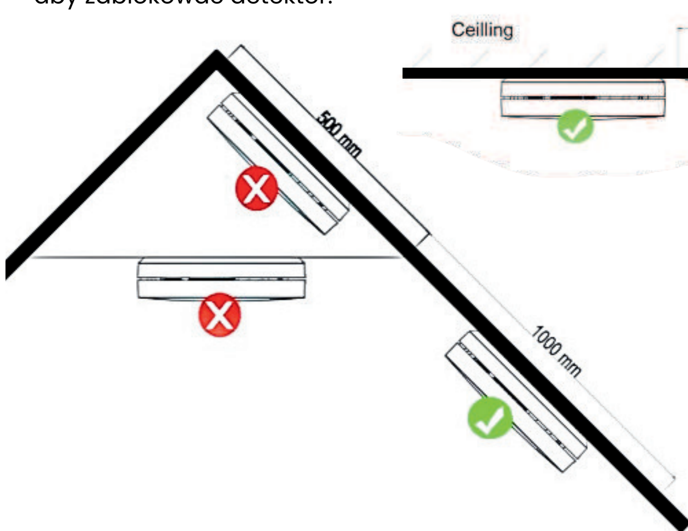
Rysunek 4: Zalecane miejsca montażu
