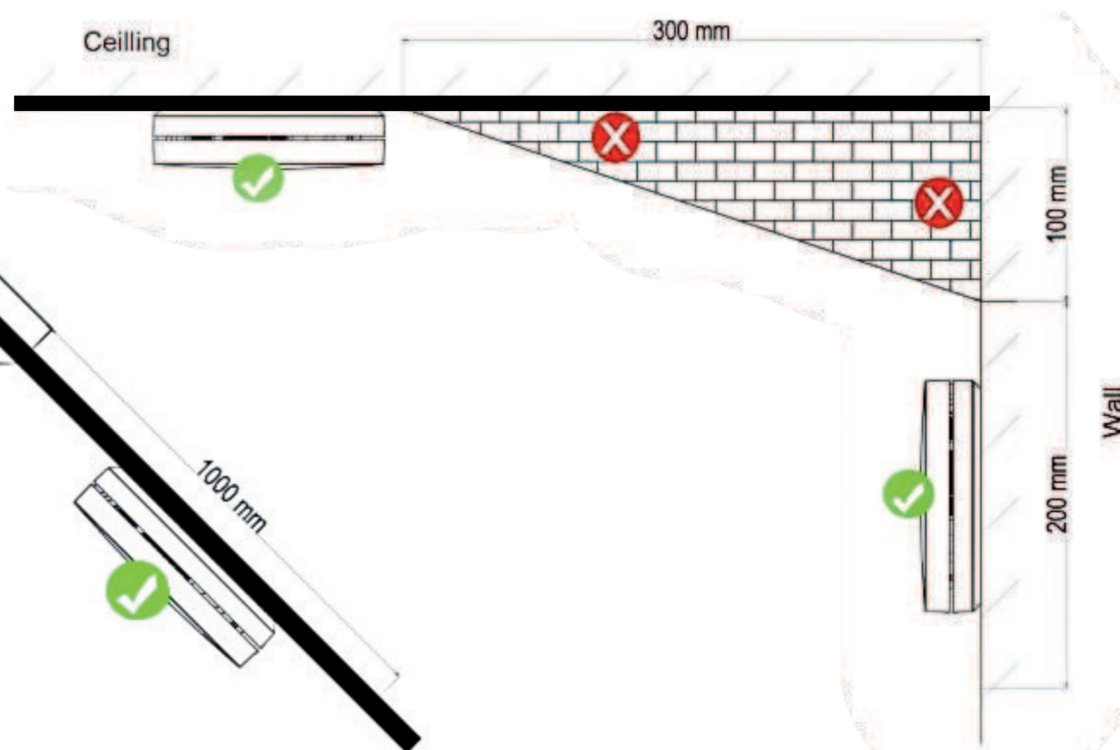
Rysunek 5: Zalecane miejsca montażu
