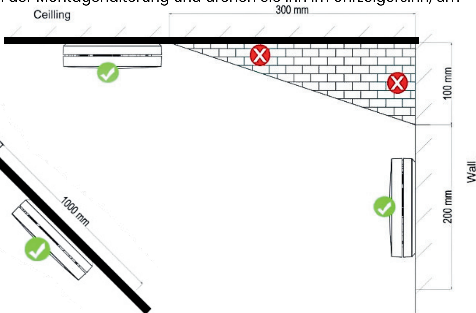
Abbildung 4: Empfohlene Montageorte
