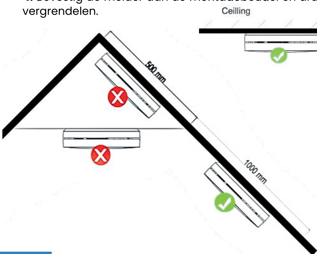
Figuur 4: Aanbevolen montagelocaties
