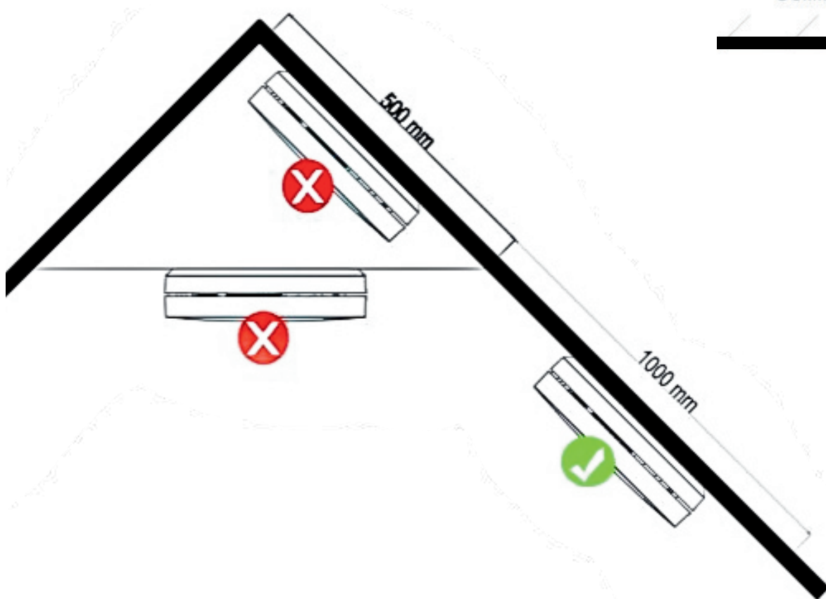
Figure 4 : Emplacements de montage recommandés
