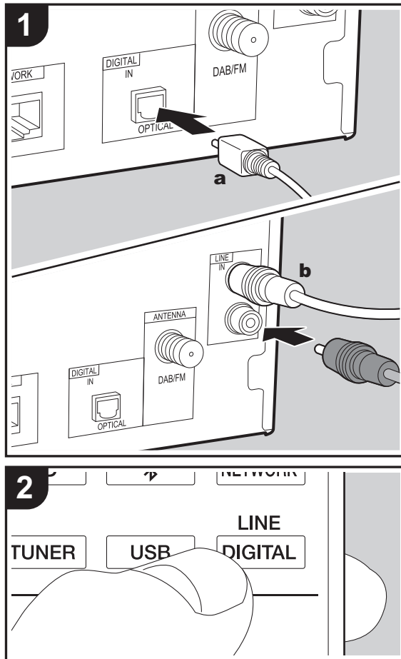
a Цифровой волоконно-оптический кабель, b Аналоговый аудиокабель
