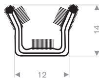
219.01.022 EPDM + textiel
