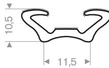
219.01.201 EPDM gevlokt
