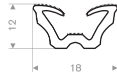
219.01.204 EPDM gevlokt
