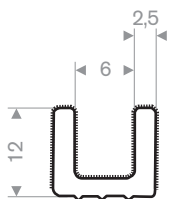
219.01.108 EPDM gevlokt
