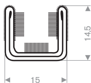
219.01.021 EPDM + textiel
