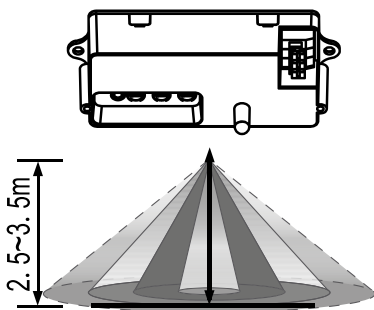
Montagehöhe: 2,5-3m
