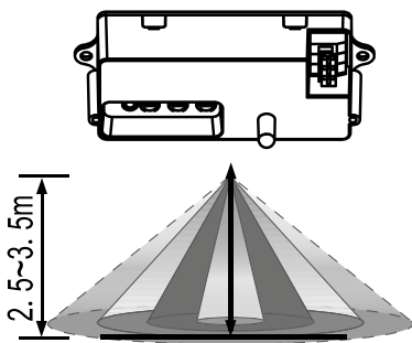
Montagehoogte: 2,5-3m
