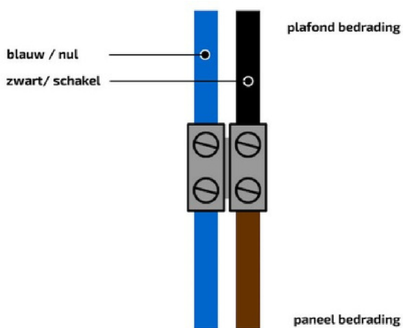
2-draads aansluiting
