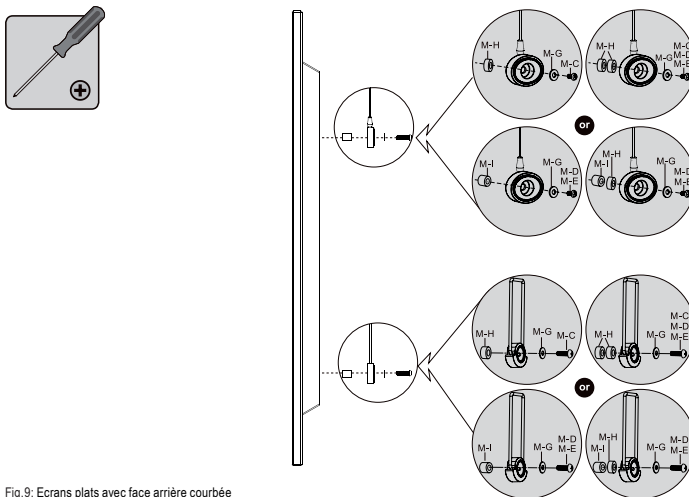
Fig. 9: Ecrans plats avec face arrière courbée
