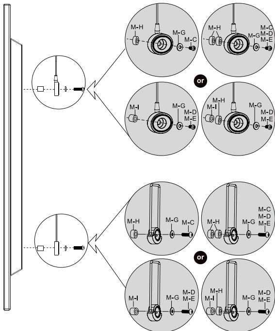
Fig. 3: Flachbildschirme mit gewölbter Rückseite
