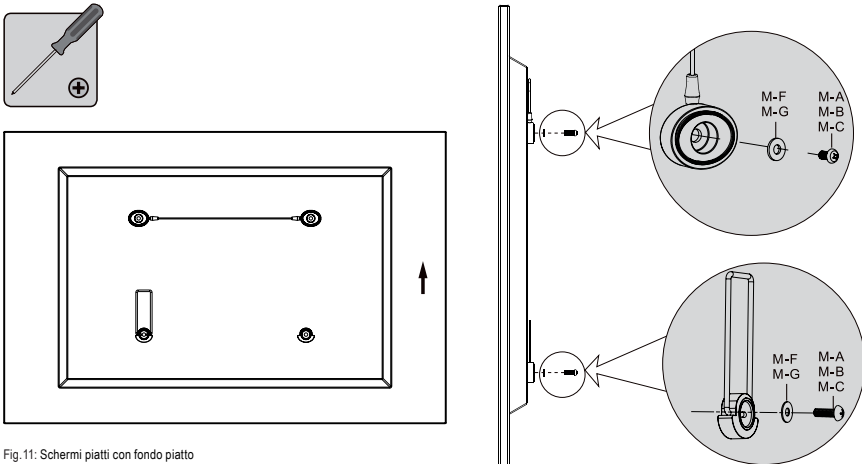
Fig. 11: Schermi piatti con fondo piatto
