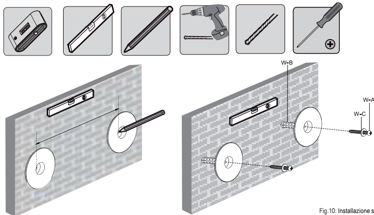
Fig.10. Installazione su parete
