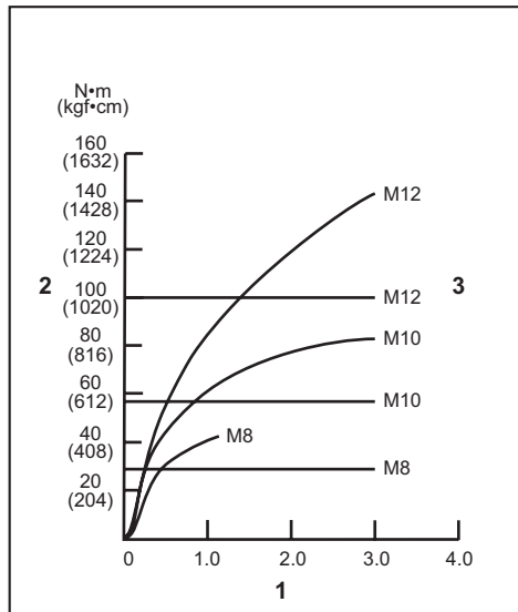
1. Tempo di serraggio (secondi) 2. Coppia di serraggio 3. Coppia di serraggio corretta corrispondente a ciascun diametro dei bulloni
