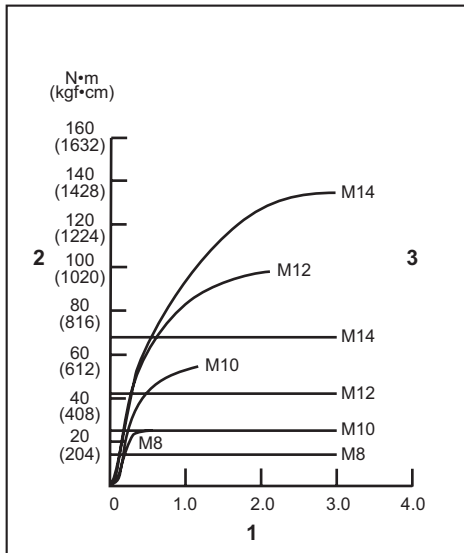
1. Aandraaitijd (seconden) 2. Aandraaimoment 3. Juiste aandraaimoment afhankelijk van de boutdiameter
