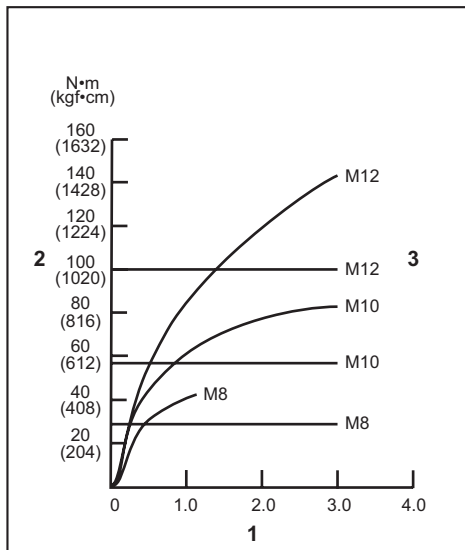
1. Tilspændingstid (sekunder) 2. Tilspændingsmoment 3. Korrekt drejningsmoment svarende til diameteren af hver bolt
