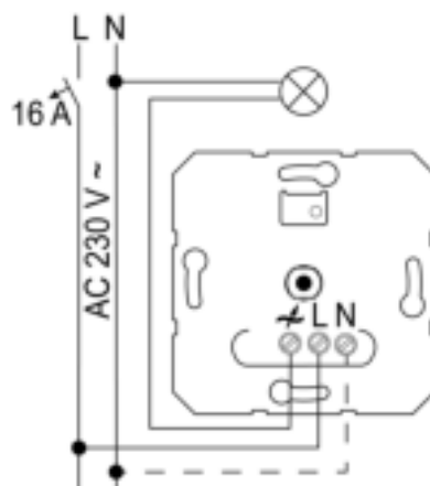
Afbeelding 3: Aansluitschema
