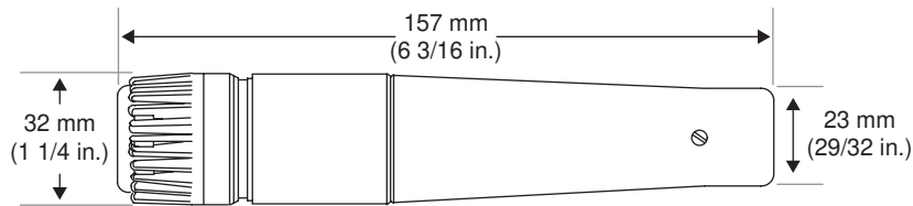
OVERALL DIMENSIONS - DIMENSIONS HORS TOUT
