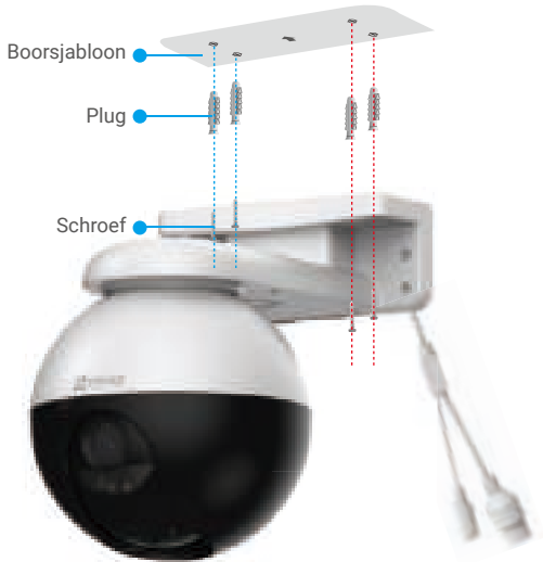
Afb. 1 Plafondmontage
