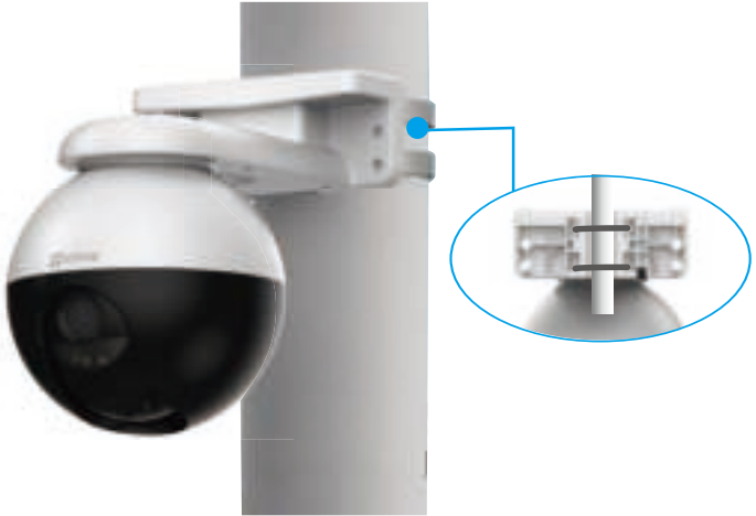
Afb. 3 Paalmontage
