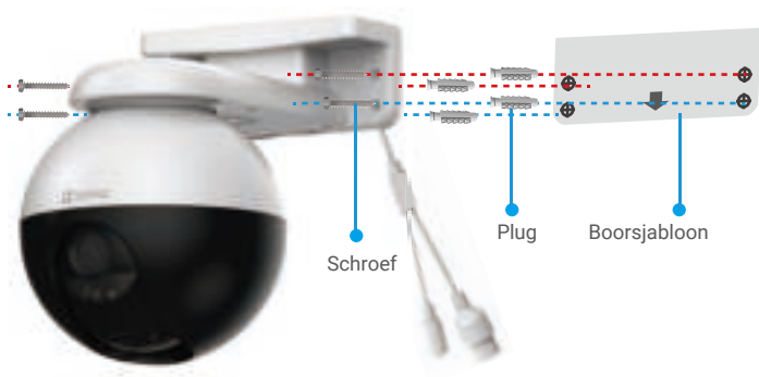
Afb. 2 Muurmontage
