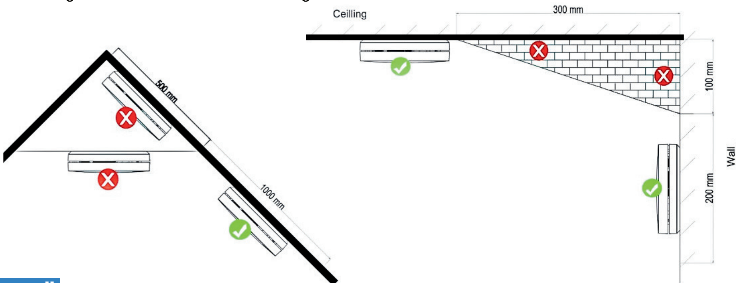
Abbildung 4: Empfohlene Montageorte
