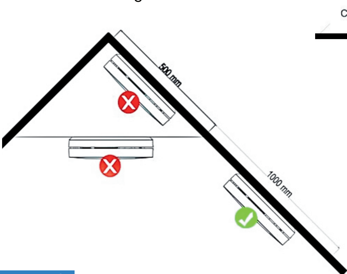
Figuur 4: Aanbevolen montagelocaties
