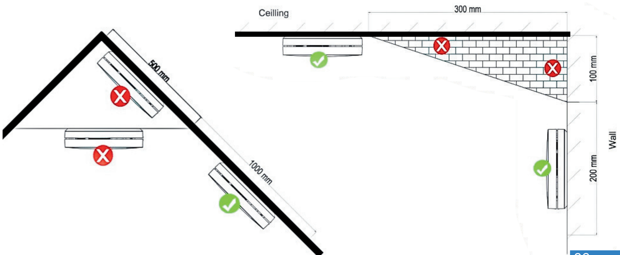
Figura 4: posizioni di montaggio consigliate
