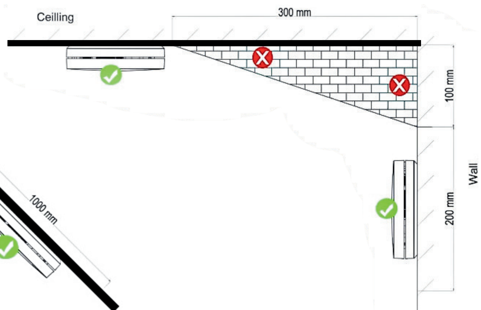
Figura 4: Ubicaciones de montaje recomendadas
