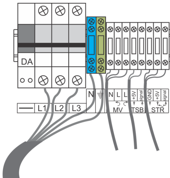
Afbeelding 9c: NOARK zekeringen
