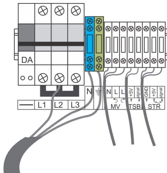
Afbeelding 9b: NOARK zekeringen
