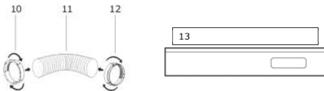
Abb. 2 Montagemaaterial Abluftschlauch
