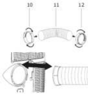
Afb. 5 Montage afvoerluchtslang
