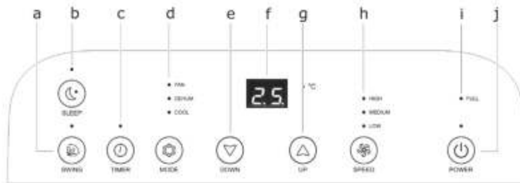
Abb. 3 Bedienblende
