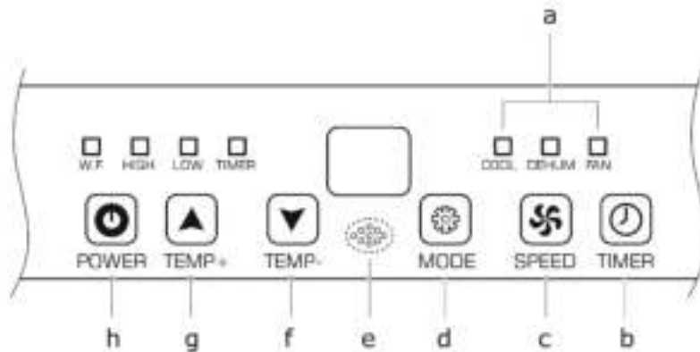
Abb. 2 Bedienblende
