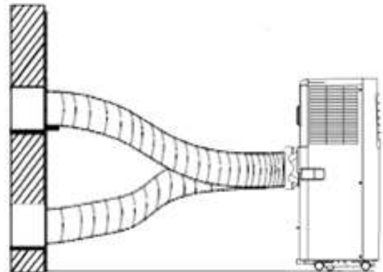
Abb. 10 Abluftschlauch: Richtiger Anschluss
