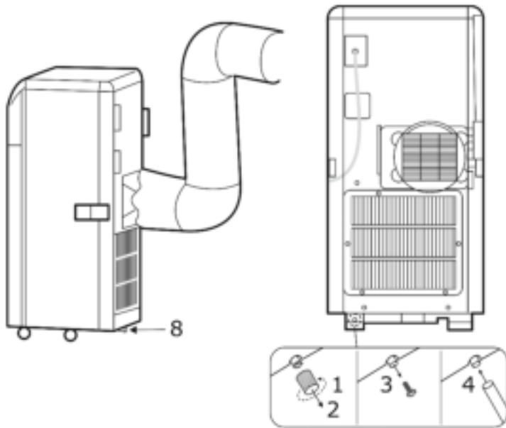
Afb. 4 Aansluiting waterafvoerslang
