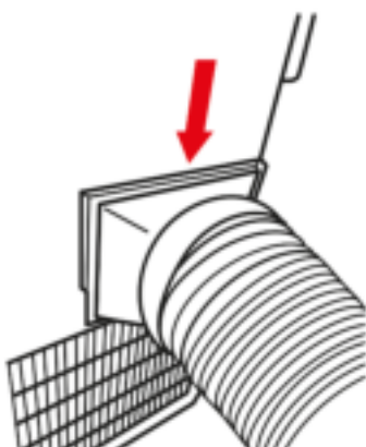
Afb. 7 Montage afvoerluchtslang
