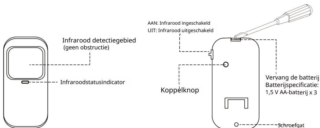
Bewegingsdetector B
