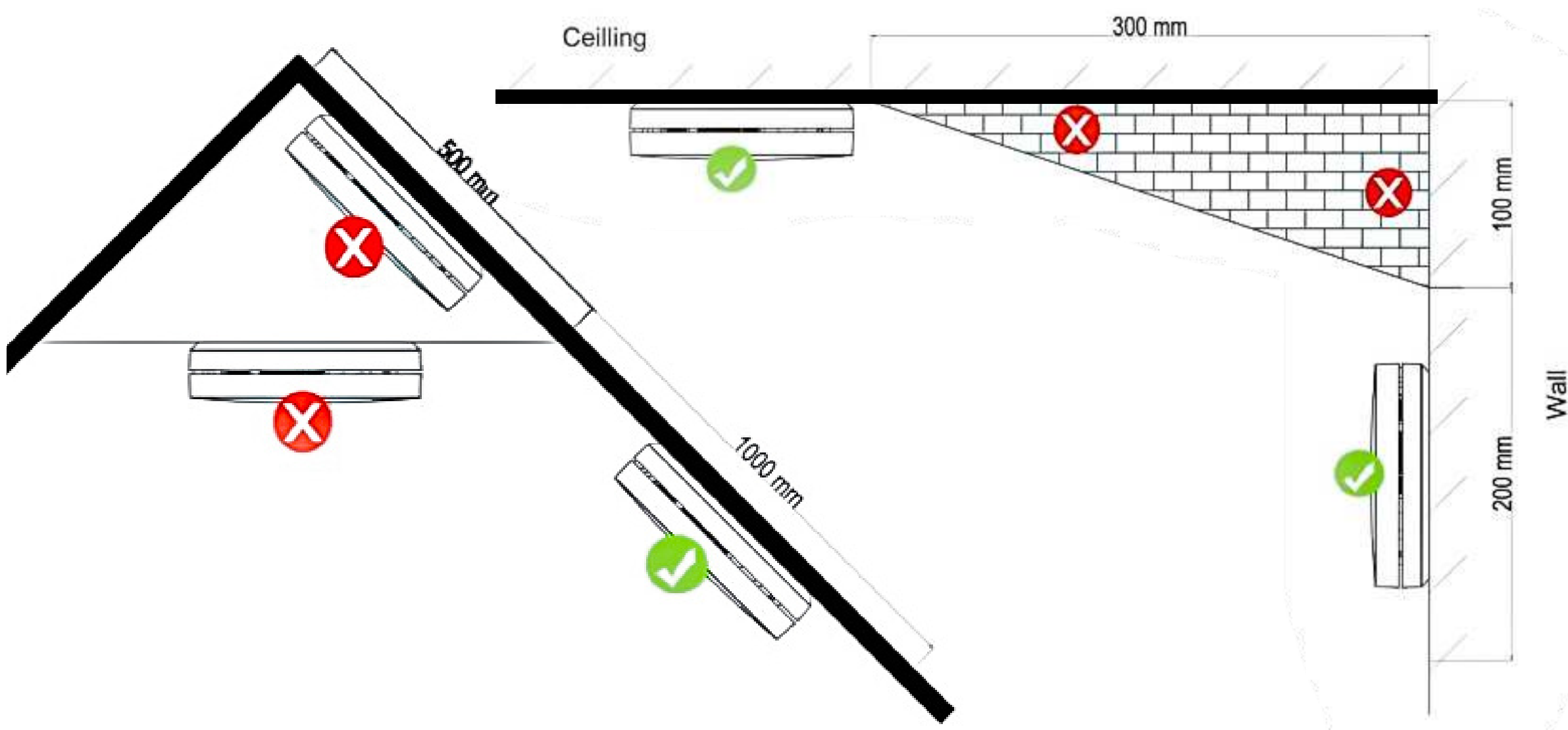
Figura 4: posizioni di montaggio consigliate
