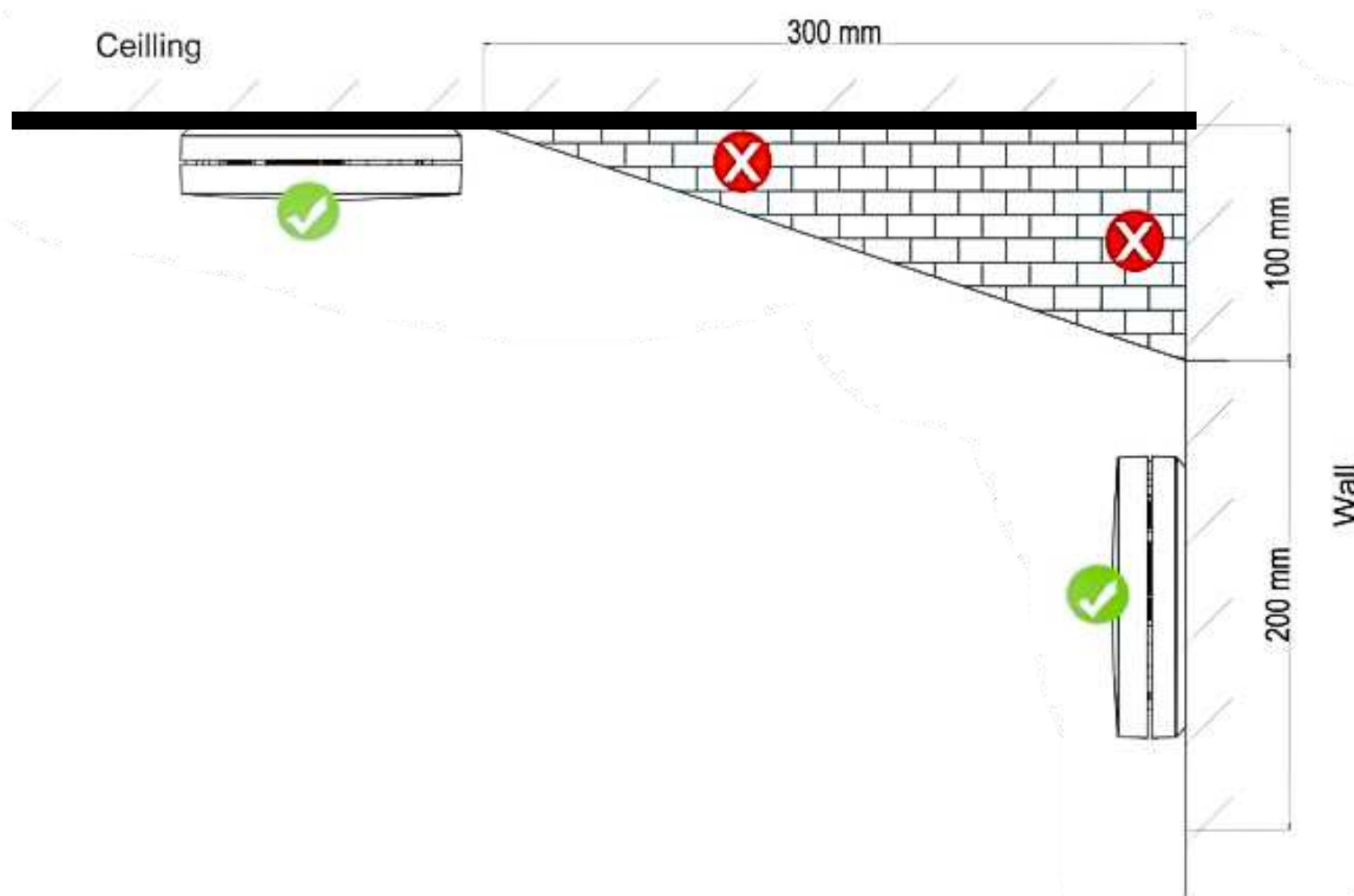
Figura 5: Ubicaciones de montaje recomendadas
