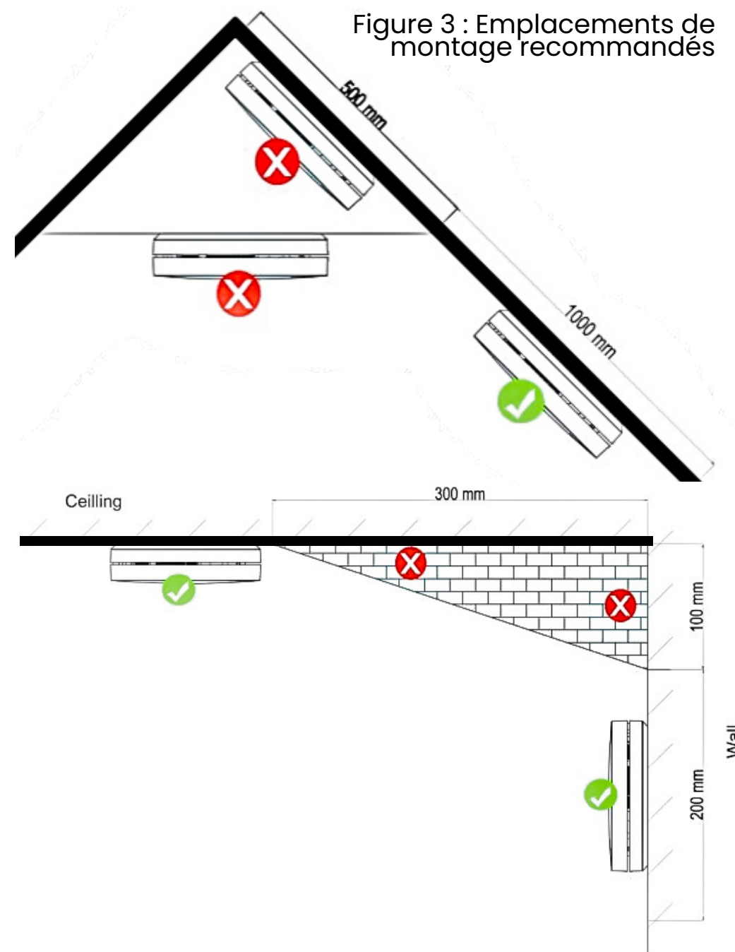
Figure 4 & 5 : Emplacements de montage recommandés
