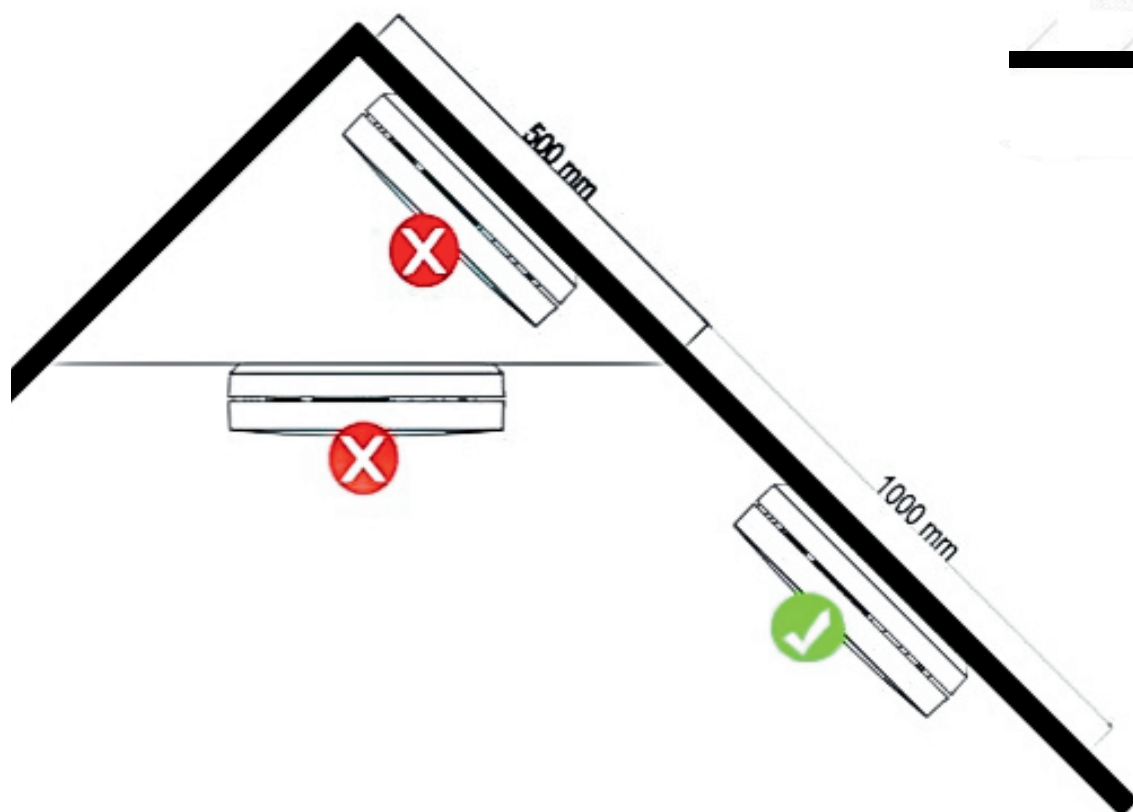
Figura 4: posizioni di montaggio consigliate
