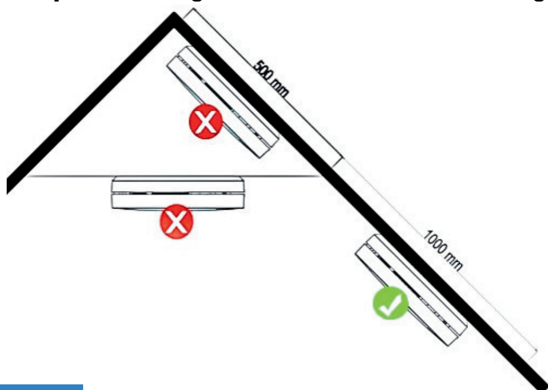
Figuur 4: Aanbevolen montagelocaties
