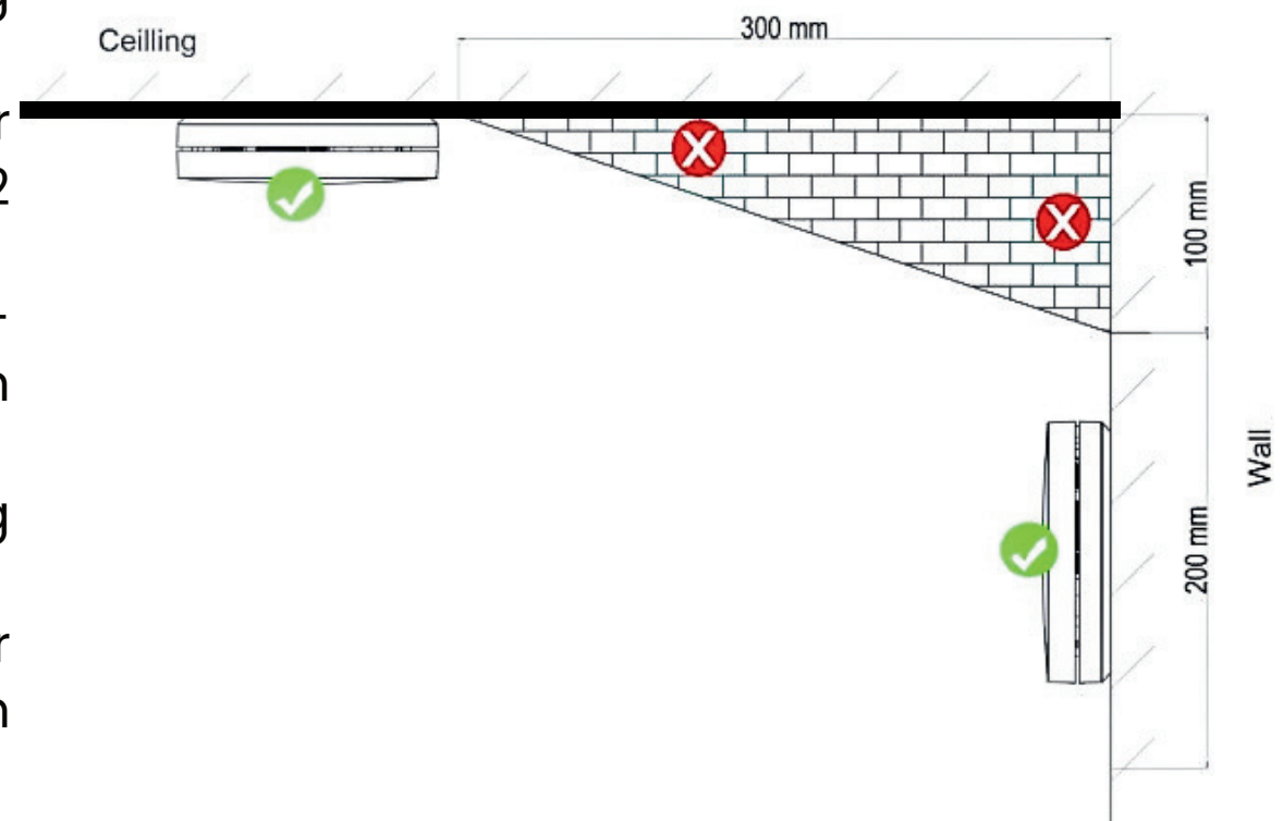
Abbildung 5: Empfohlene Montageorte
