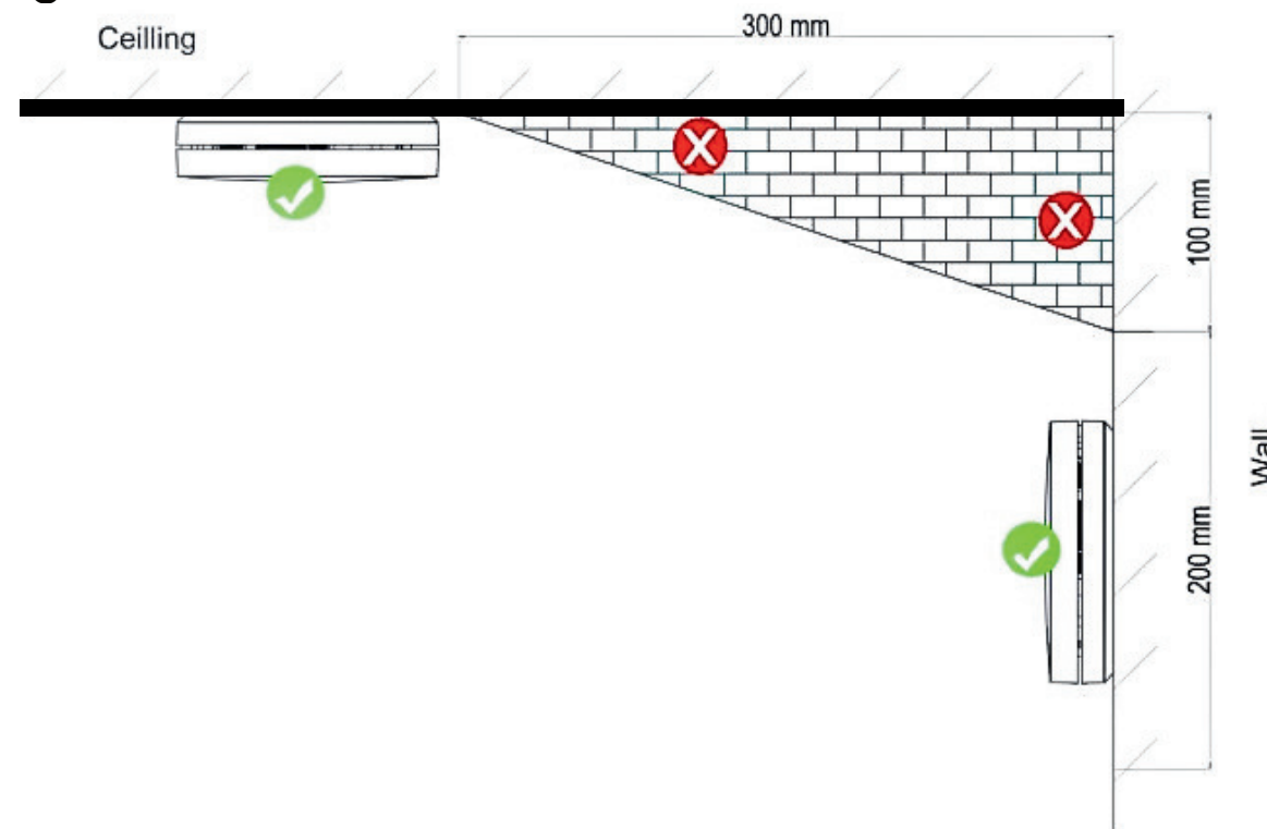
Figuur 5: Aanbevolen montagelocaties
