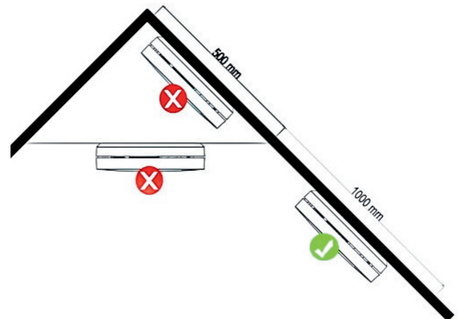
Abbildung 4: Empfohlene Montageorte
