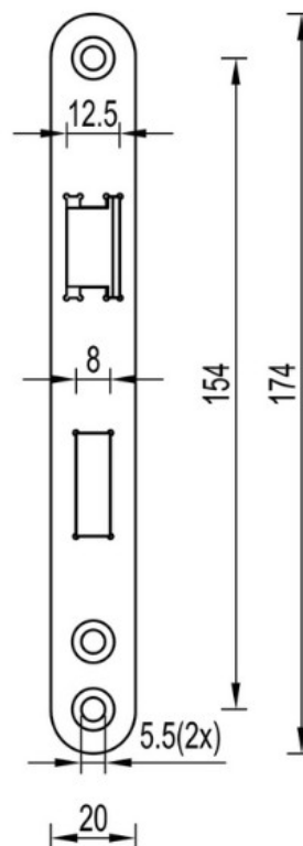
VOORAANZICHT (SLOTPLAAT)
