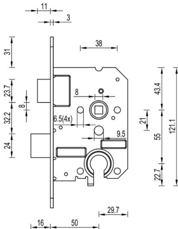
ZIJAANZICHT (SLOTKAST)
