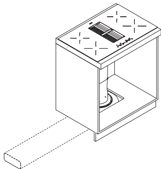
uitvoering 1, linkeruitlaat
