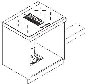
uitvoering 3, rechteruitlaat
