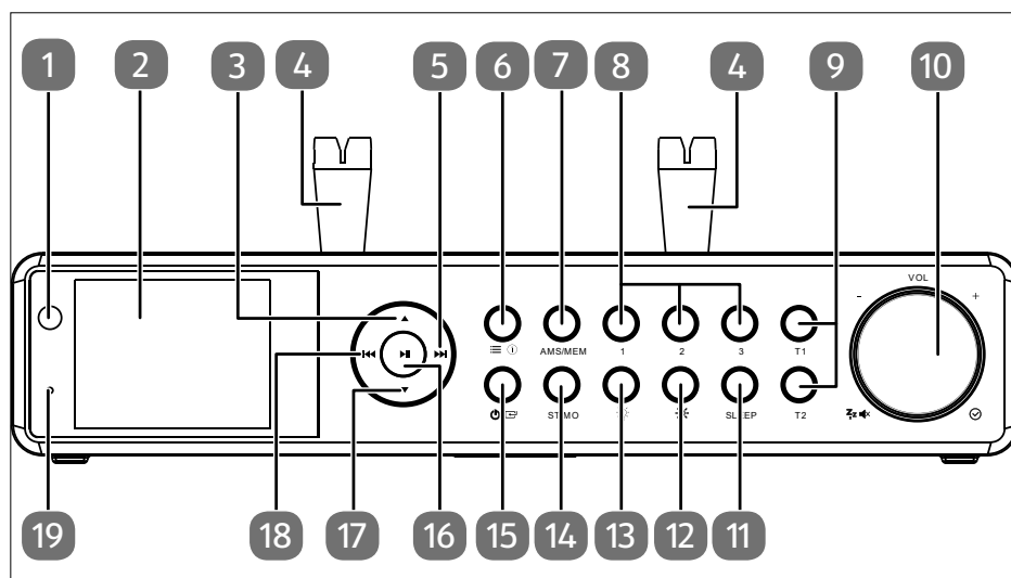
Fig. 1 – Vista delantera
