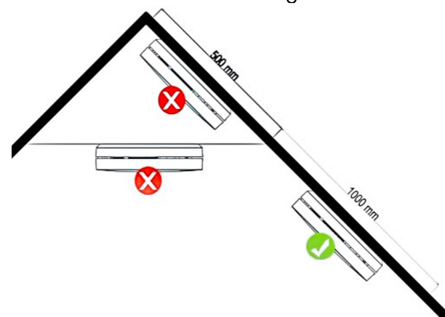
Figure 4 : Emplacements de montage recommandés
