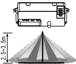
Montagehoogte: 2,5-3m
