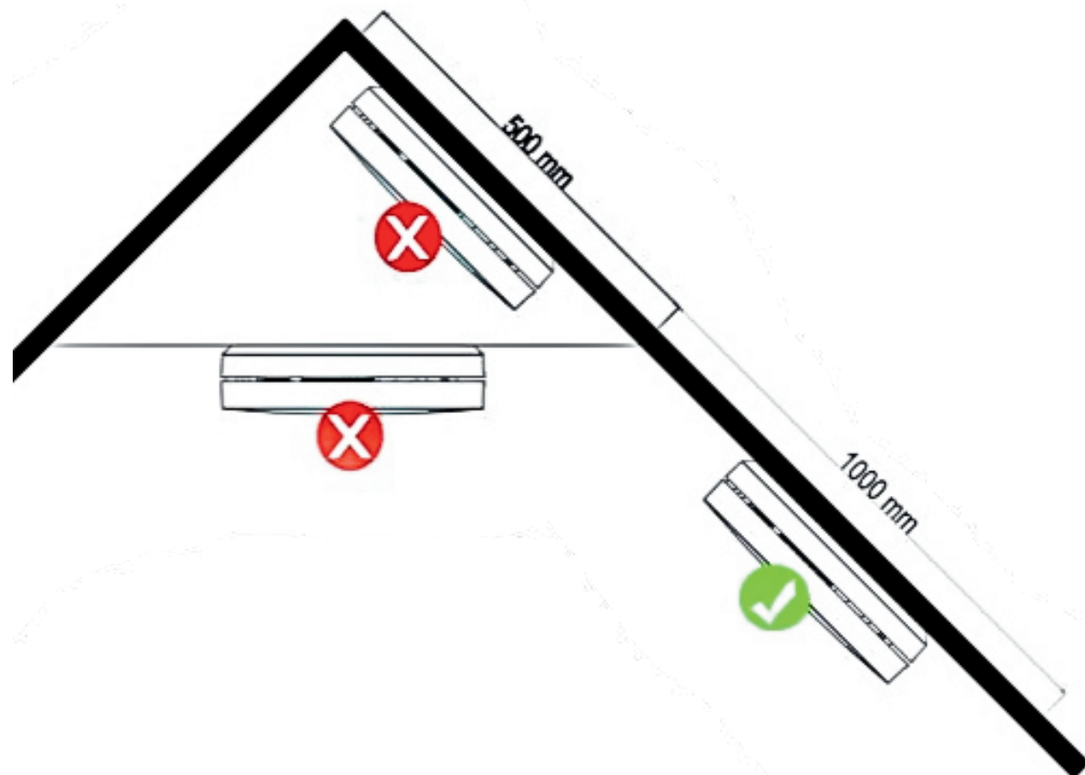
Figura 4: Ubicaciones de montaje recomendadas
