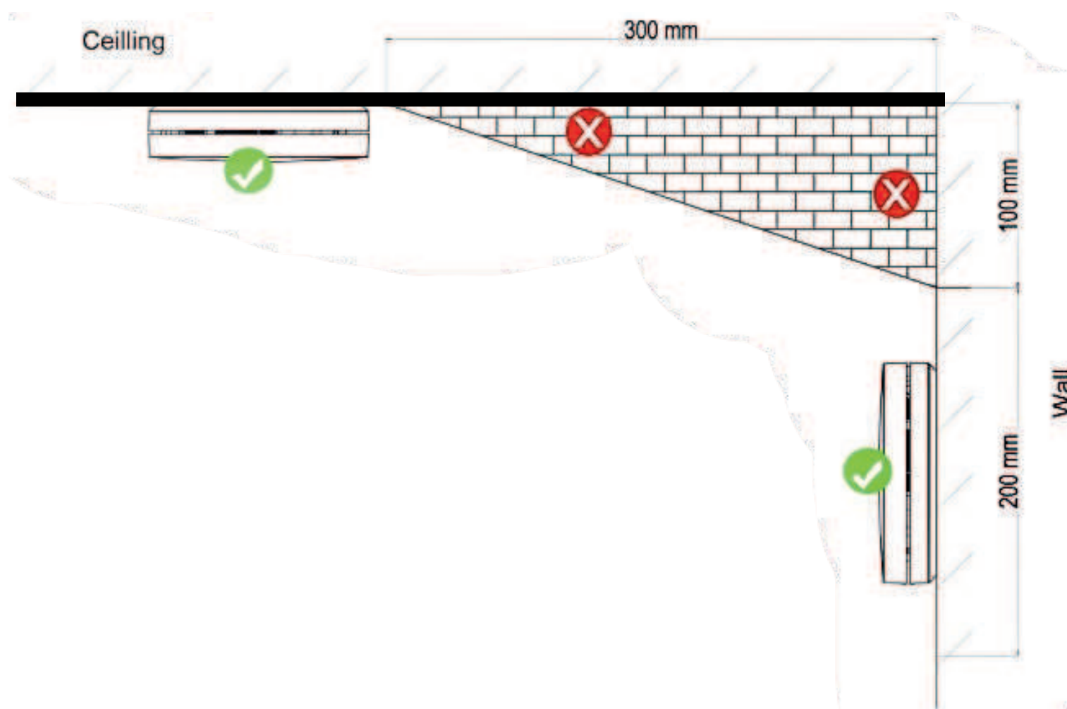
Figura 5: Ubicaciones de montaje recomendadas
