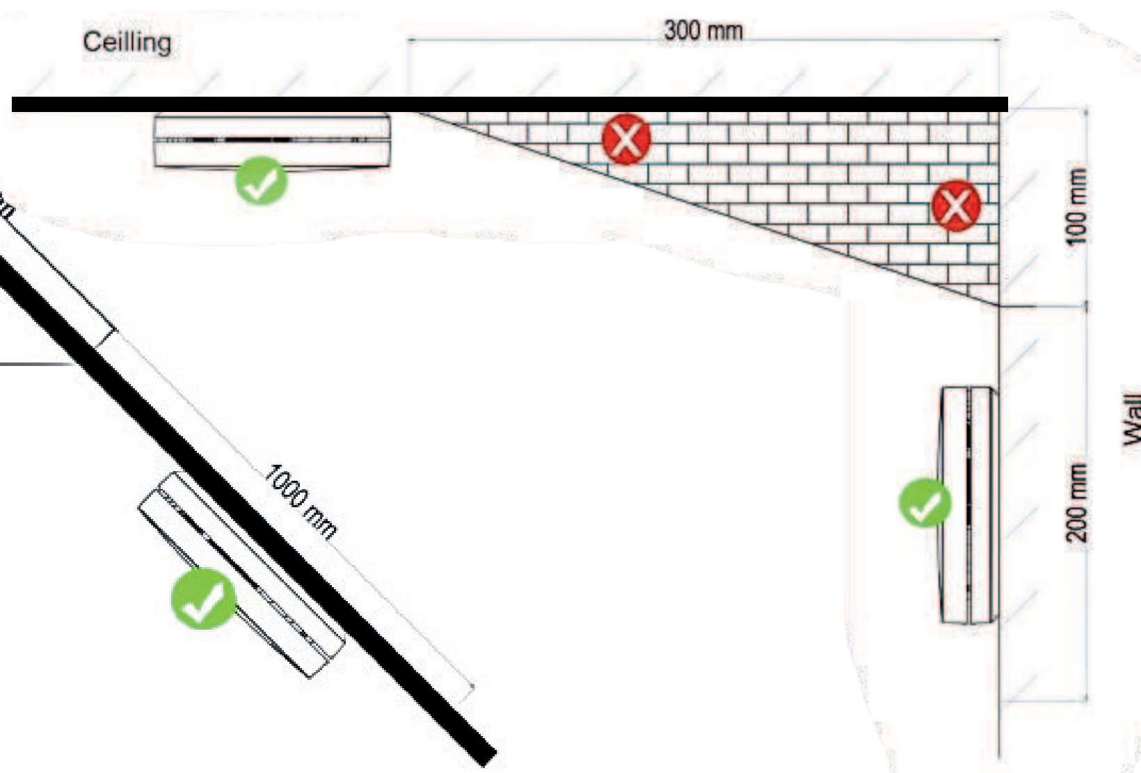
Figura 4: posizioni di montaggio consigliate
