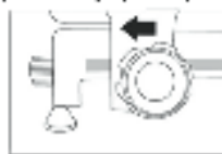
3) Ustaw pokrętło na żądaną grubość krojenia. Przesuń pokrętło do lewej strony aż do zatrzymania.
