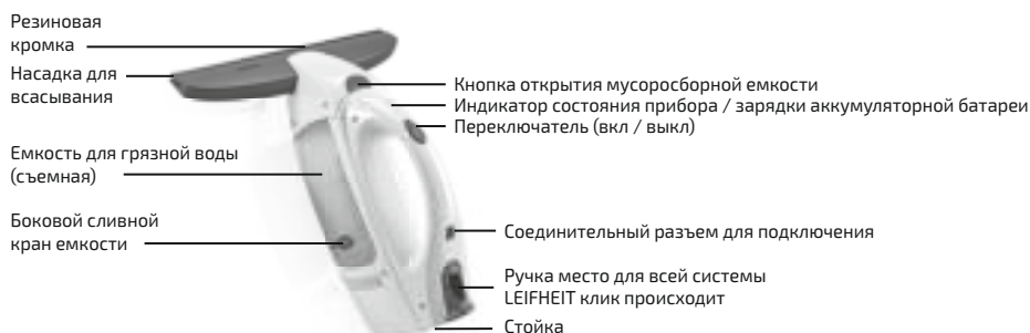
Рисунок 2: Элементы управления оконным пылесосом
