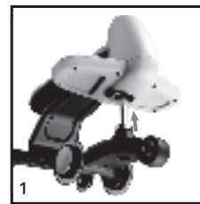
Abbildung 1: Die Vorderradbaugruppe (Teil 4) in das Loch der Karosserie (Teil 1) montieren.
