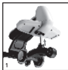
Figura 1: Instale el montaje de la rueda delantera (pieza 4) en el orificio de la carrocería (pieza 1).
