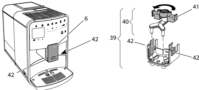
Afb. 22: Toevoer draaien
