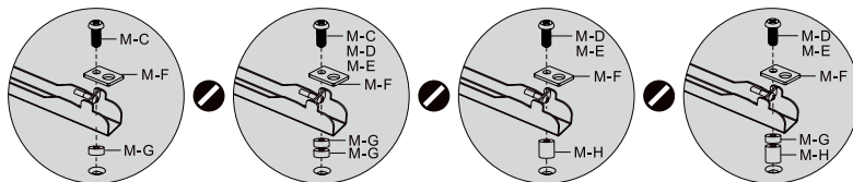
Fig.20: Schermi piatti con fondo curvo
