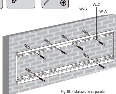
Fig.18: Installazione su parete
