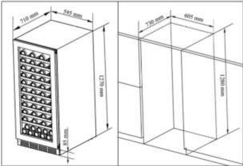
Model D104T bovenaanzicht
