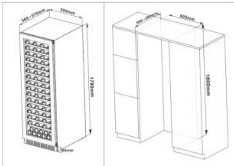
Model D92T bovenaanzicht
