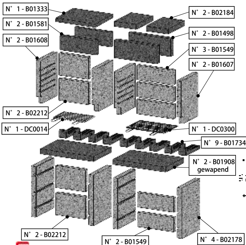
Onderdelen overzicht
