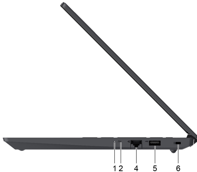
Figuur 10. Rechterkant—Lenovo V14 G4 IRU, Lenovo V14 G4 IAH en Lenovo V14 G4 ABP
