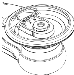
7. Suojalaipan tai välilaitan kanssa käytettävä kokoonpano.
