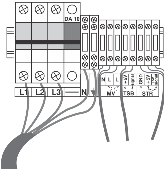
Schema van de verbindende klem en aansluiting van het apparaat op driefasige stroomvoorziening
