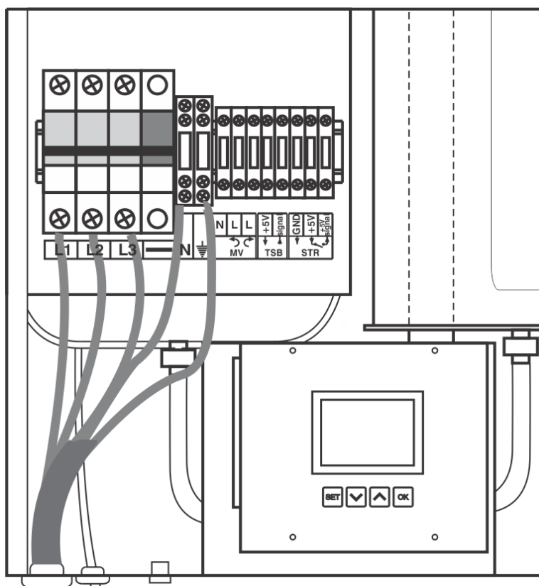
Afbeelding 7: aansluitschema van de stroomkabel
