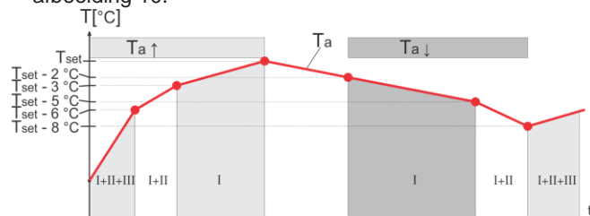
Afbeelding 10: Schakel de elementen in en uit
